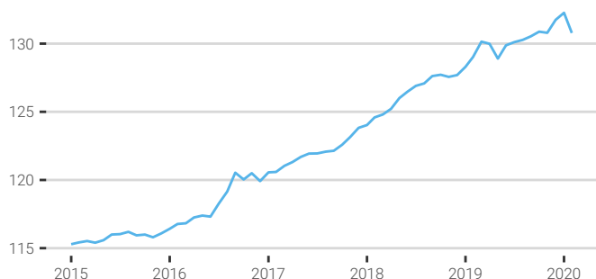
Fig. 1. Evolution de l'indice emploi salarié marchand
