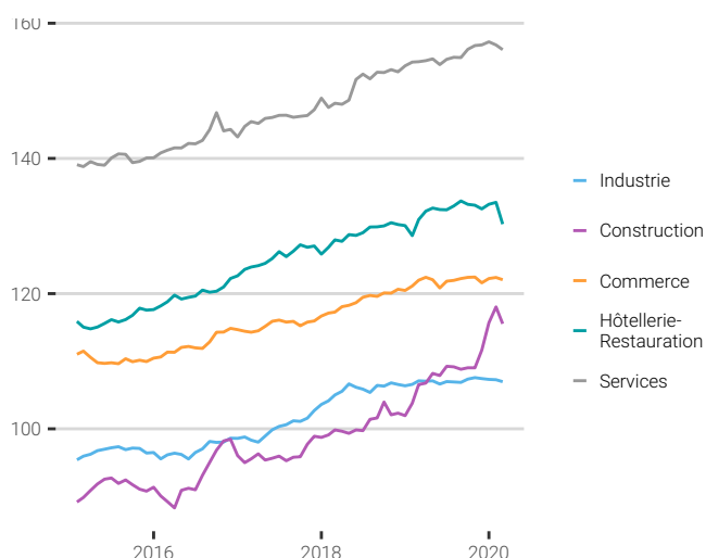
Fig. 2. Evolution des indices par secteur d'activités
